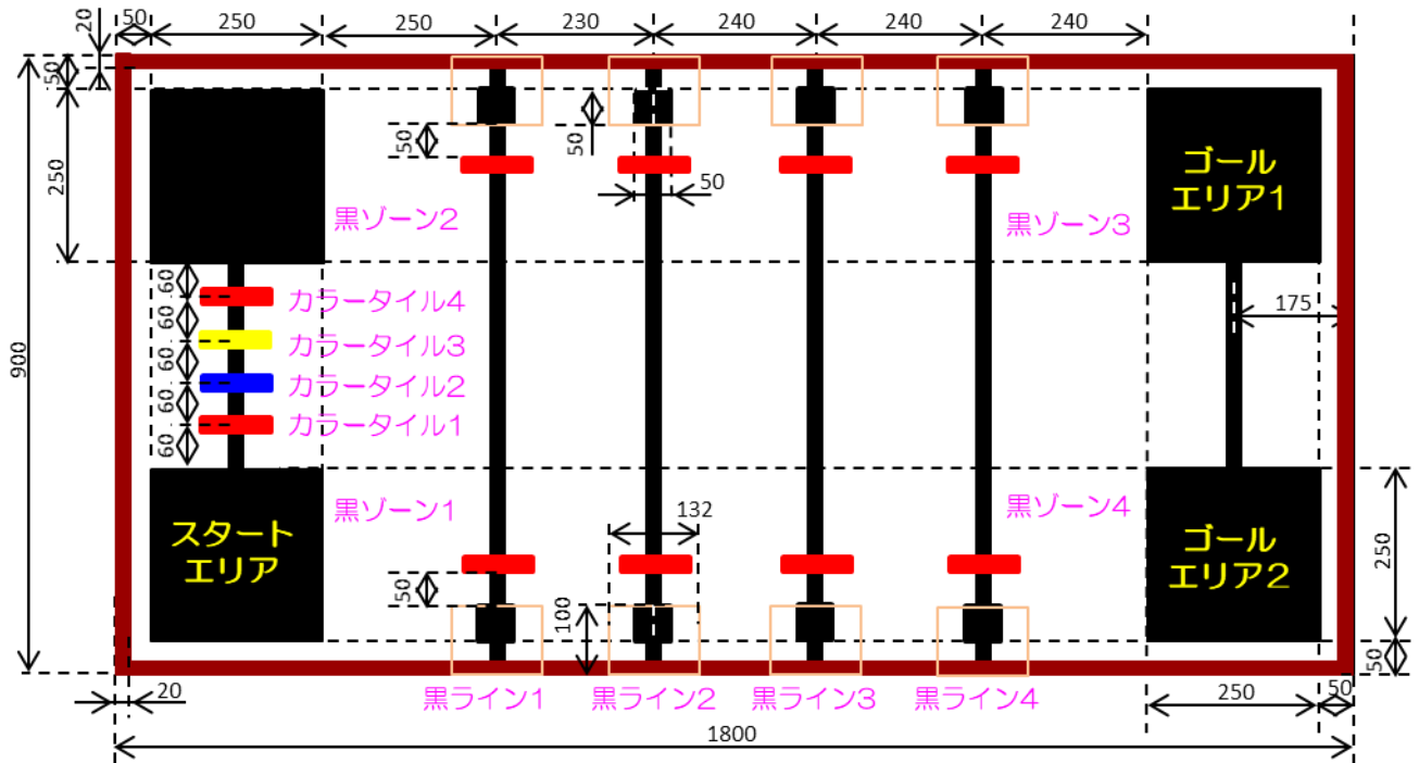
図 1 WRO Japan 2021 ミドル フィールド (カラータイルは例)
